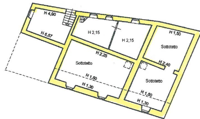
Piano Primo
